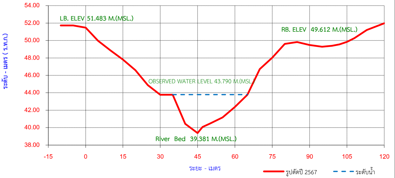
รูปตัดขวางลำน้ำ ปีน้ำ 2567 สถานี N.22 แม่น้ำแควน้อย อ.วัดโบสถ์ จ.พิษณุโลก
